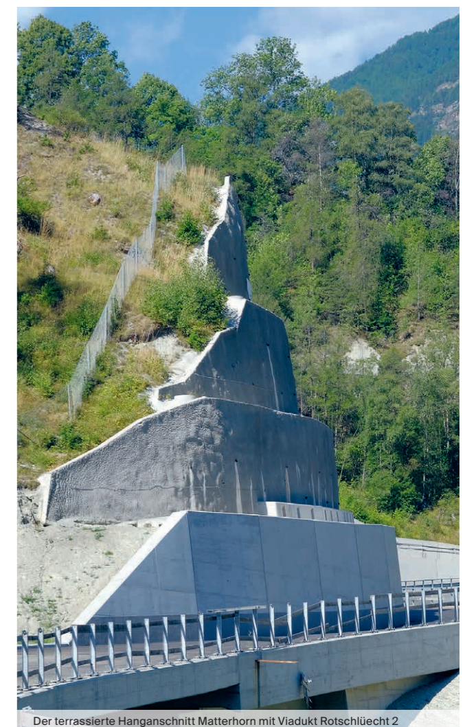
Der terrassierte Hanganschnitt Matterhorn mit Viadukt Rotschlüecht 2
